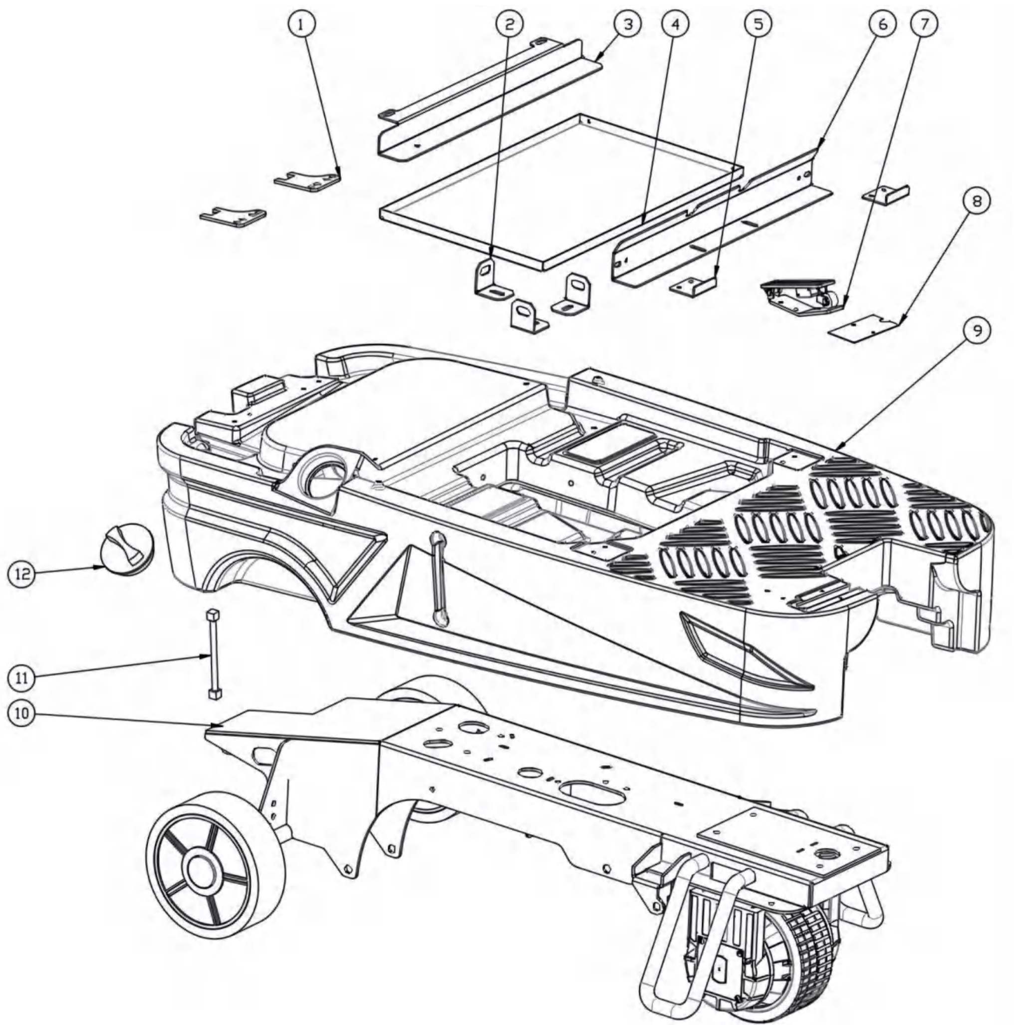
Fig. 8 -FRONT GROUP
